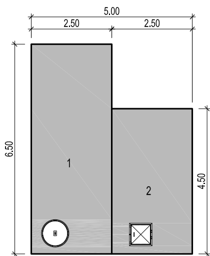
PIANTA COPERTURE
