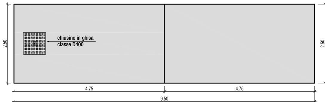
PIANTA COPERTURA
