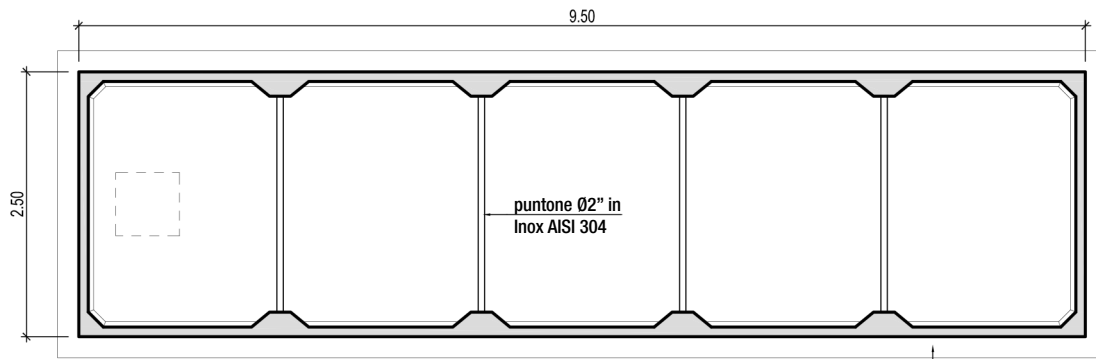
PIANTA
